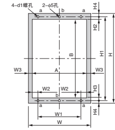
面板加工图1
