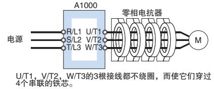
接线图b
