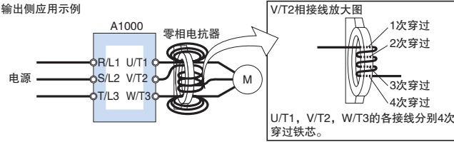
接线图a
