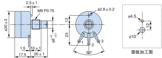
外形尺寸 mm
